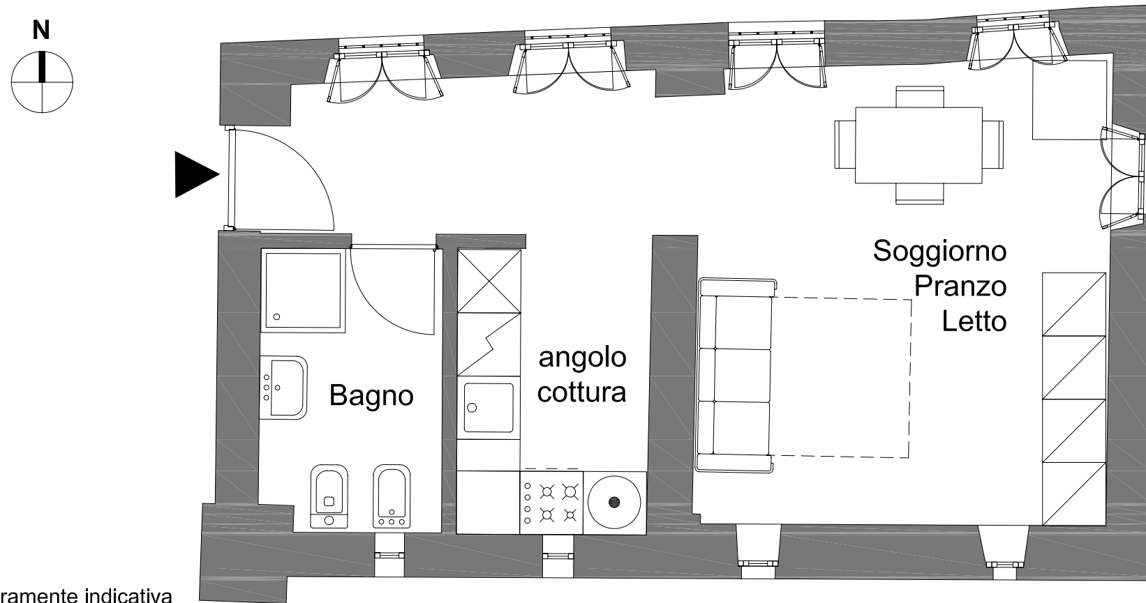
PLANIMETRIA GENERALE
